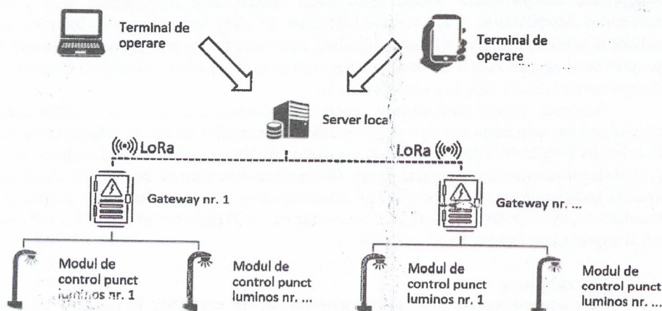
(Schema principiu de functionare)
