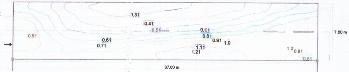
Observator 1: Valoarea de întreținere, densitatea luminii cu carosabil uscat [ \text{cd}/\text{m}^2 ] (Linii Isolux)
